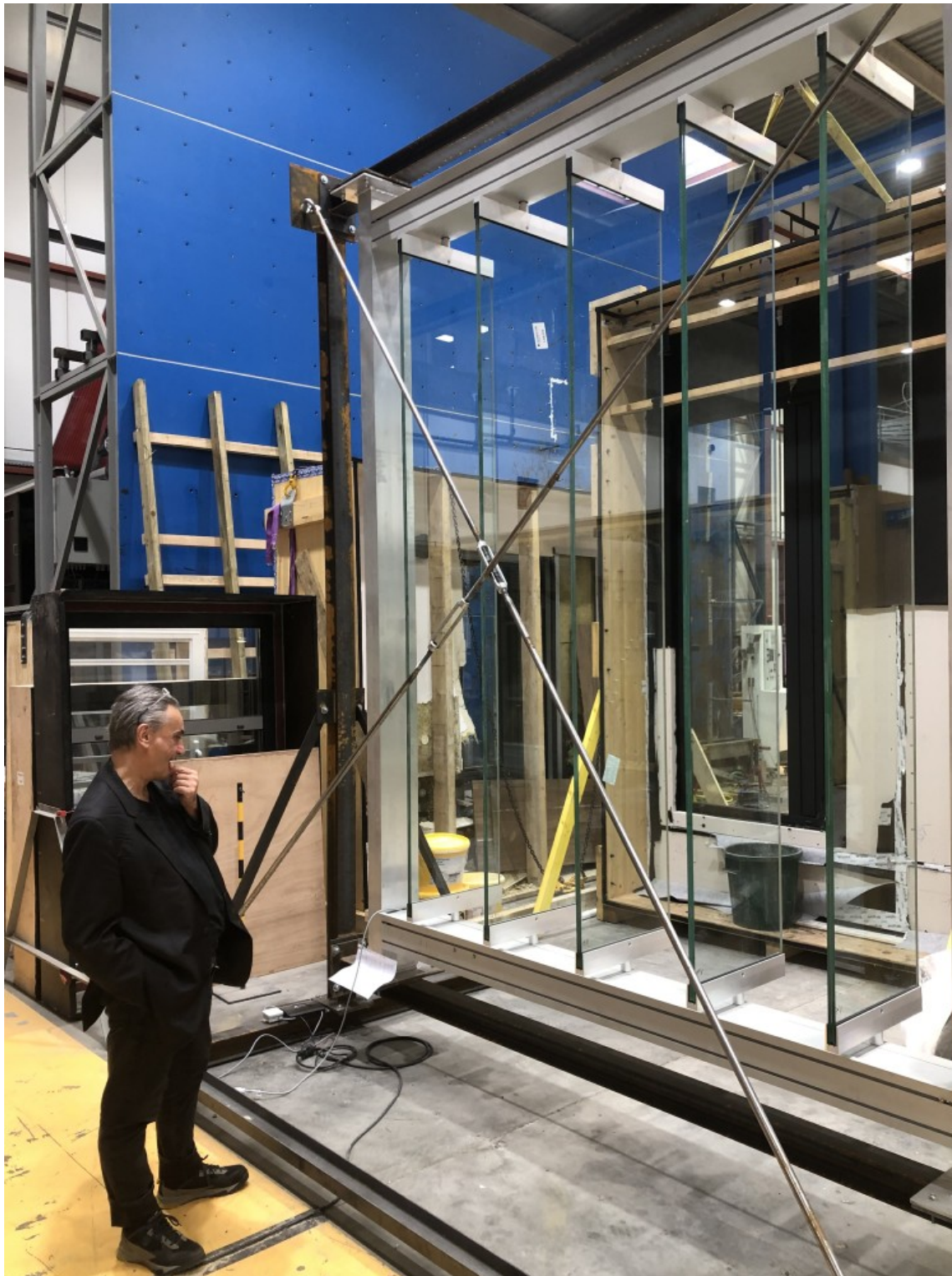
atex: surfaçade en lames de verre mobiles pour la restructuration du centre jean sarrailh du crous de paris entreprise kingspan atex obtenu en juillet 2024 (cstb)
